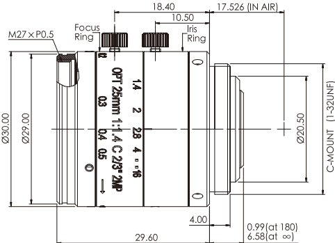
6.OPT-C2514-2M
