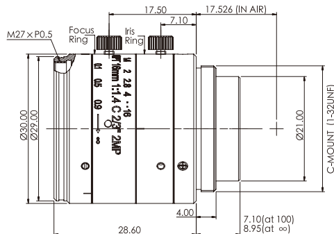
5.OPT-C1614-2M
