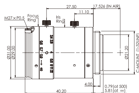
8.OPT-C5024-2M
