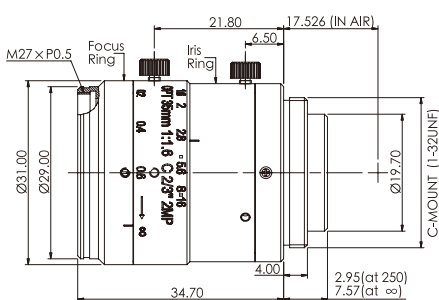
7.OPT-C3516-2M
