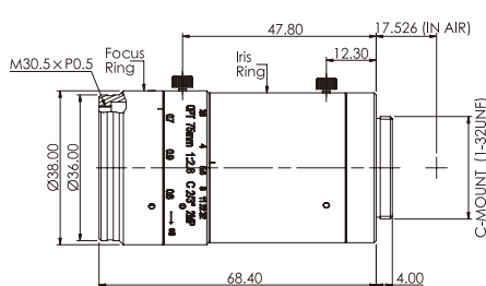
9.OPT-C7528-2M
