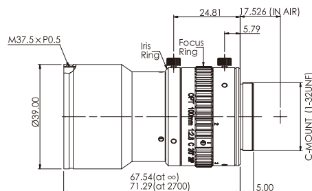
10.OPT-C10028-2M
