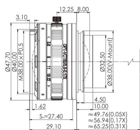
9.OPT-VCT60/5.6-0.17X
