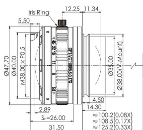
11.OPT-VCT100/5.6-0.17X
