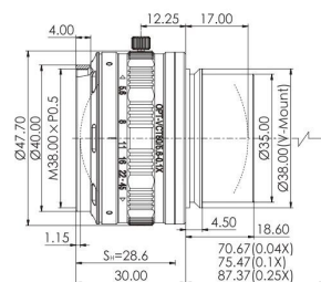
10.OPT-VCT80/5.6-0.1X
