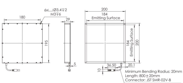
7. OPT-IFLA200200
