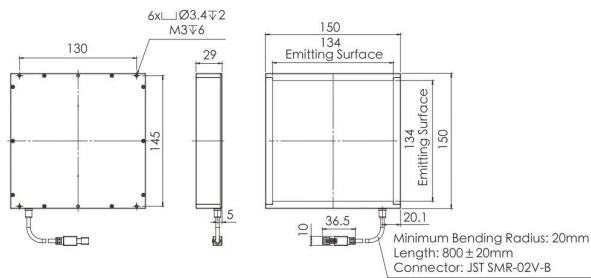
5. OPT-IFLA150150
