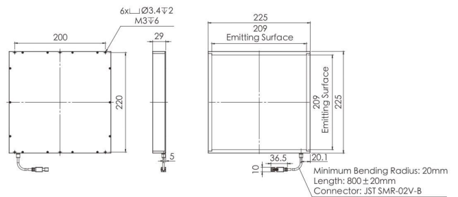
8. OPT-IFLA225225
