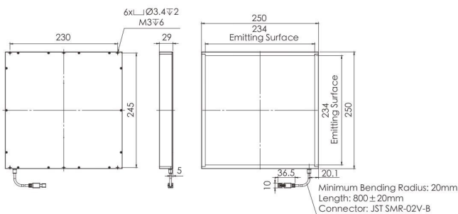
9. OPT-IFLA250250
