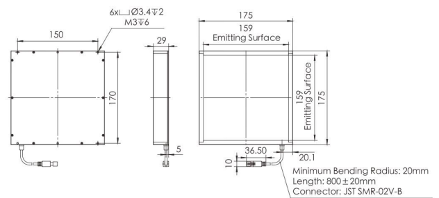
6. OPT-IFLA175175
